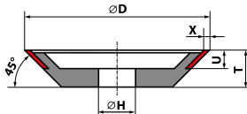
Typ 12V9 Ściernica diamentowa i borazonowa 12V9 - D \times T \times X \times U \times H
