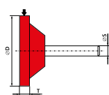
Typ 5201 Ściernica trzpieniowa płaska ze stożkowym wzmocnieniem 5201 - D \times T \times S
