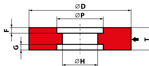
SPOSÓB OZNACZANIA 7 - D × T × H - P...F...G...
