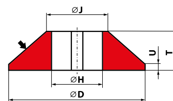
SPOSÓB OZNACZANIA 301 - D/J × T/U × H
