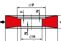
Typ 25 Ściernica z wybraniem stożkowo - walcowym i stożkowym z drugiej strony 25 - D/K × T/N × H - P... F...
