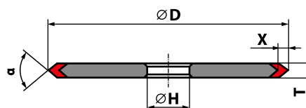
SPOSÓB OZNACZANIA 1EE1- \alpha - D \times T \times X \times H
