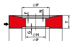
Typ 24 Ściernica z wybraniem stożkowo - walcowym i walcowym z drugiej strony 24 - D × T/N × H - P... F... G...
