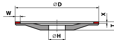
SPOSÓB OZNACZANIA 12A2PA- D × T-X × W × X × H
