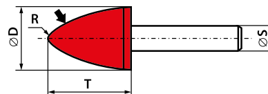
SPOSÓB OZNACZANIA 5220 - D × T × S - R
