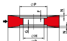
Typ 26 Ściernica z dwustronnym wybraniem stożkowo - walcowym 26 - D × T/N × H - P... F... G...
