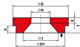
Typ 3801 Ściernica do młynków pulpy 3801 - D / J × T / U × H - nr rys
