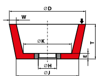
Typ 1114 Ściernica garnkowa stożkowa z wkładką gwintową 1114 - D/J × T × H - W...E...K...
