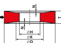
Typ 21 Ściernica z dwustronnym wybraniem stożkowym 21 - D/K × T/N × H
