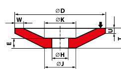
Typ 12 Ściernica talerzowa 12 - D/J × T/U × H - W...E...K...
