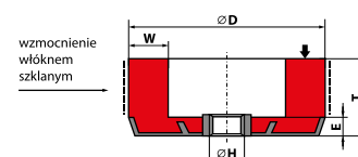
Typ 6004 Ściernica garnkowa walcowa z wkładką gwintową 6004 - D × T × H - W...E...
