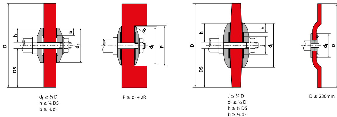
System montażu z zastosowaniem kołnierza mocujących dla ściernic z małym otworem centralnym Q \leq 0,20
