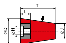
Typ 17 Ściernica stożkowa ścięta z wkładką gwintową 17 - D/J × T/U - H × L
