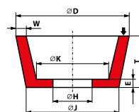
Typ 11 Ściernica garnkowa stożkowa 11 - D/J × T × H - W...E...K...
