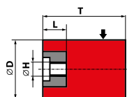
Typ 18 Ściernica walcowa z wkładką gwintową 18 - D × T - H × L
