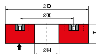
36 - D × T × H - ... - nr rysunku
