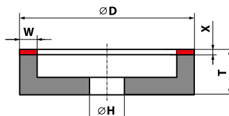
6A2 - D × T-X × W × X × H
