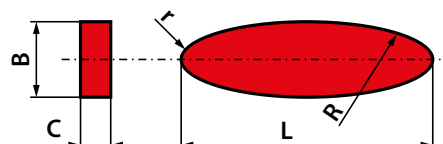
SPOSÓB OZNACZANIA 9050 - B × C × L - R...r...
