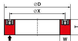
Typ 37 Ściernica pierścieniowa z wkładkami gwintowymi 37 - D \times T - W... - nr rys.
