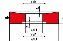
Typ 22 Ściernica z wybraniem stożkowym i walcowym z drugiej strony 22 - D/K × T/N × H - P... F...
