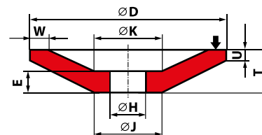
SPOSÓB OZNACZANIA 12 - D/J × T/U × H - W...E...K...
