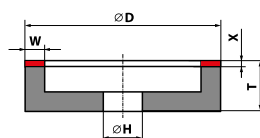
Typ 6A2 Ściernica diamentowa i borazonowa 6A2 - D \times T \times X \times W \times X \times H
