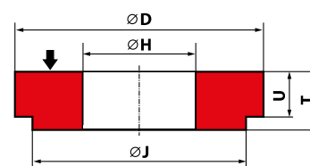
35X - D × T × H - ... - nr rysunku
