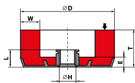
Typ 6005 Ściernica garnkowa walcowa z wkładką gwintową 6005 - D × T × H/L - W...E...
