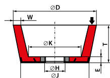
Typ 1113 Ściernica garnkowa stożkowa z wkładką gwintową 1113 - D/J × T × H - W...E...K...
