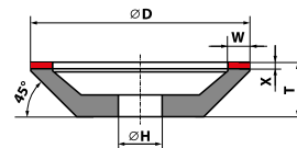
Typ 12A2-45 Ściernica diamentowa i borazonowa 12A2-45 - D \times T \times X \times W \times X \times H
