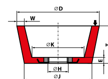
Typ 1112 Ściernica garnkowa stożkowa z wkładką gwintową 1112 - D/J × T × H - W...E...K...
