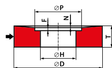
Typ 23 Ściernica z jednostronnym wybraniem stożkowo - walcowym 23 - D × T/N × H - P... F...
