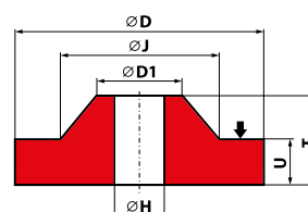
3802 - D/J × T/U × H - ... - V - nr rysunku
