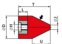
Typ 19 Ściernica walcowo - stożkowa z wkładką gwintową 19 - D/J × T/U - H × L
