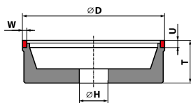
Typ 6A9 Ściernica diamentowa i borazonowa 6A9 - D \times T \times X \times U \times H
