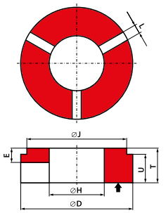
Typ 3504 Ściernica tarczowa z nacięciami jednostronnie odsadzona 3504 - D / J \times T / U / E \times H - L...n - ilość nacięć
