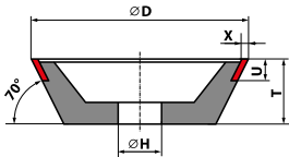
Typ 11V9 Ściernica diamentowa i borazonowa 11V9 - D \times T \times X \times U \times H
