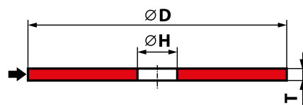
SPOSÓB OZNACZANIA 41 - D × T × H
