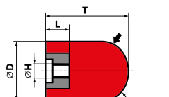
Typ 18R Ściernica walcowa zaokrąglona z wkładką gwintową 18R - D × T - H × L
