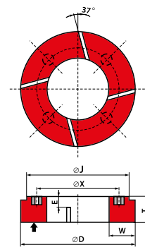
Typ 3701 Ściernica pierścieniowa z wkładkami gwintowymi odsadzeniem i nacięciami 3701 - D \times T - W... - nr rys.
