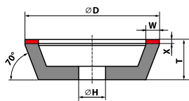
Typ 11A2 Ściernica diamentowa i borazonowa 11A2 - D \times T \times X \times W \times X \times H
