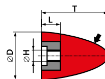
Typ 16 Ściernica stożkowa zaokrąglona z wkładką gwintową 16 - D × T - H × L
