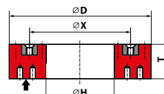
Typ 3601 Ściernica tarczowa z wkładkami gwintowymi i perforacją 3601 - D \times T \times H - nr rys.
