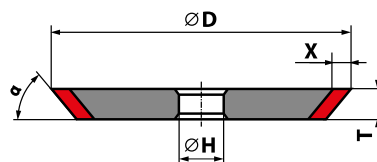
SPOSÓB OZNACZANIA 1V1- \alpha - D \times T \times X \times H
