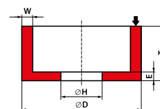
6 - D \times T \times H - W \dots E \dots
