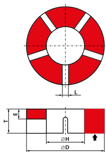
Typ 3501 Ściernica tarczowa z nacięciami 3501 - D \times T / E \times H - L...n - ilość nacięć
