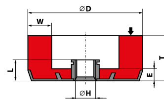
6005 - D × T × H/L - W...E...
